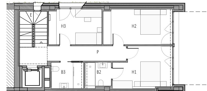
PLANTA PRIMERA
