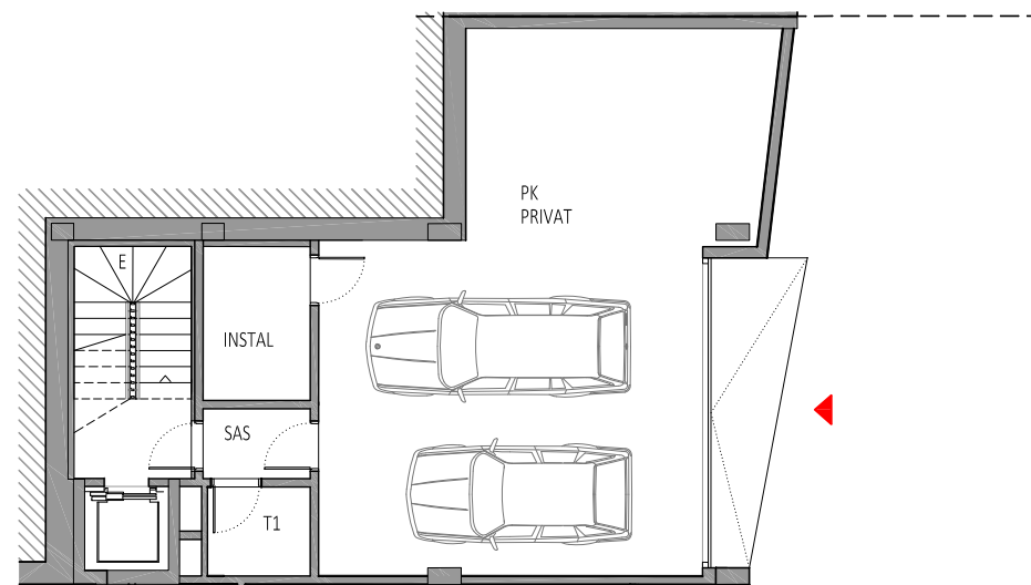
PLANTA SOTERRANI
